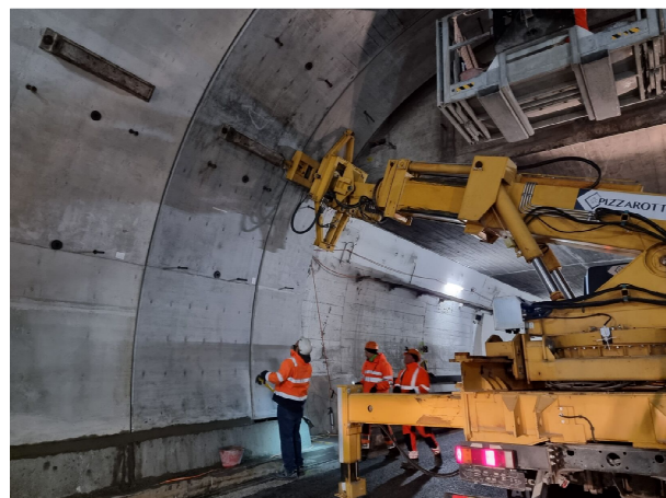
Posa dell'ultimo elemento di controanello
