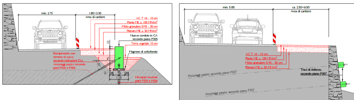
Figura 2: Dettaglio cordolo retro-ancorato a sinistra e rinforzo muro esistente in pietra a destra
