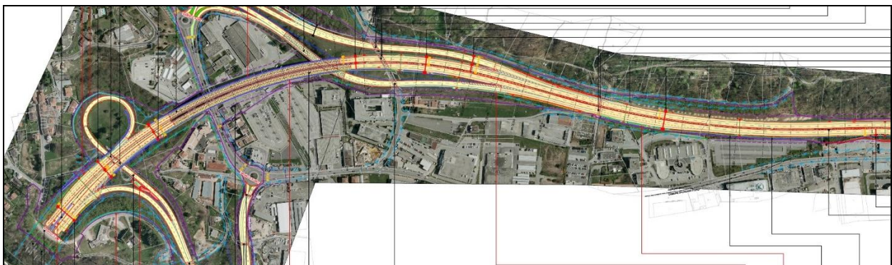
Tratto a cielo aperto: planimetria d'intervento
