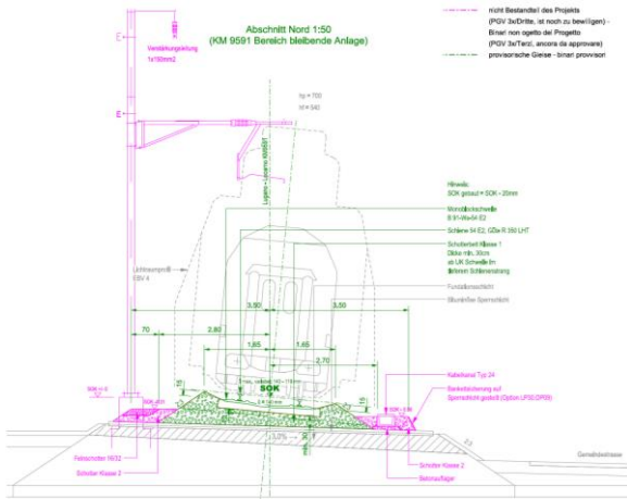
Sezione tipo binario provvisorio (ARGE AMC)
