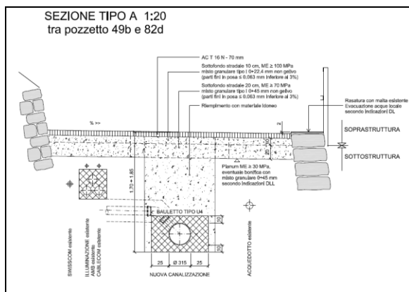
Sezione tipo nuovo collettore acque miste al Gaggio
