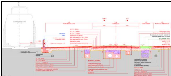
Via Basilea - Sezione tipo stradale e infrastrutture
