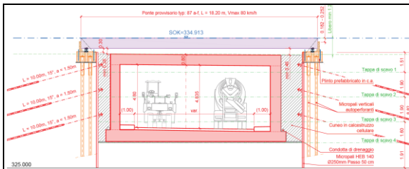
Sottopasso Genzana - Opere provvisoriale
