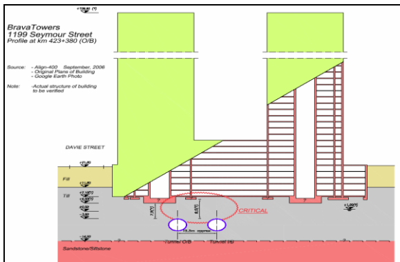
Attraversamento Brava Towers - Analisi dei rischi
