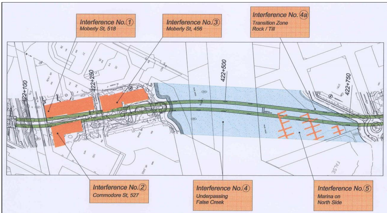
Attraversamento False Creek - Interferenze principali
