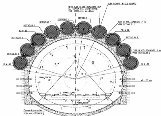
Lotto 8A: Sezione C1 - Microtunnel - Studio varianti
