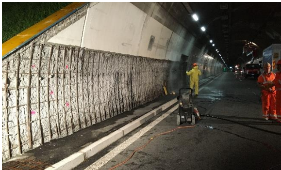
Galleria di Gentilino: riprofilatura paramenti
