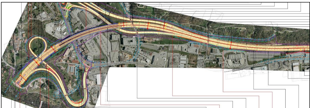
Tratto a cielo aperto: planimetria d'intervento (Consorzio TraCia)
