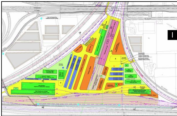
Lavori lungo la linea FFS Giubiasco - S. Antonino Lotti 714 / 741 / 751 / 771 - AlpTransit Nodo di Camorino
