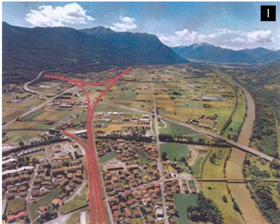
Lavori lungo la linea FFS Giubiasco - S. Antonino Lotti 714 / 741 / 751 / 771 - AlpTransit Nodo di Camorino
