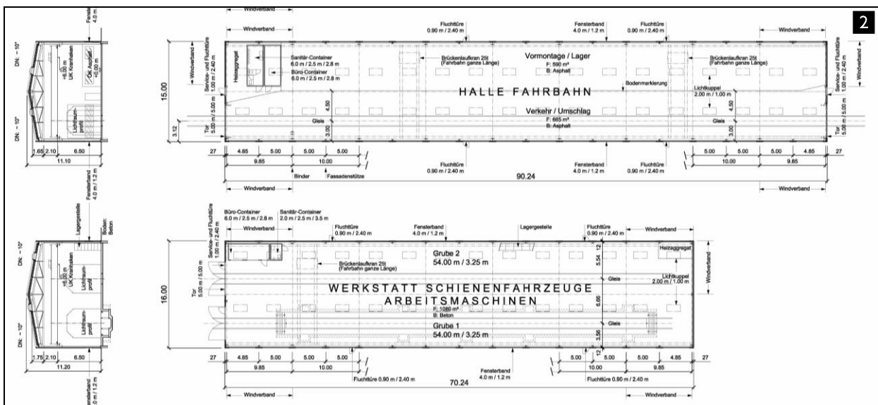
Tecnica Ferroviaria, Einbau und Logistik - AlpTransit Galleria di base del Ceneri
