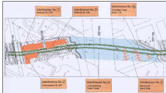
Attraversamento False Creek - Interferenze principali
