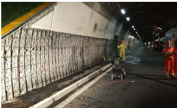
Galleria di Gentilino: riprofilatura paramenti
