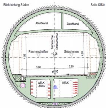
Profilo normale galleria in roccia (Consorzio IG G2)
