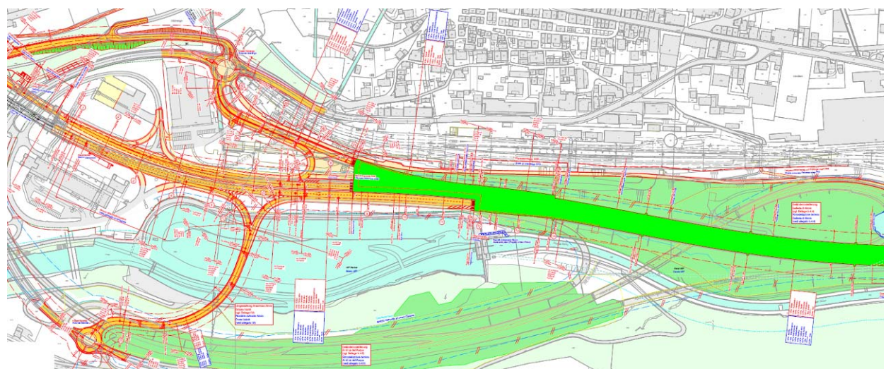
Planimetria con particolare della situazione al portale sud (Consorzio IG G2)
