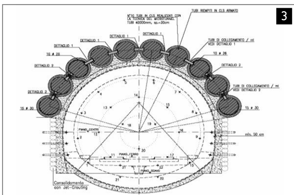
Lotto 8A: Sezione C1 - Microtunnel - Studio varianti
